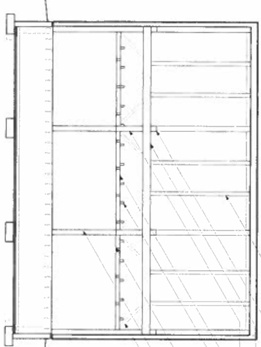
20 LONGITUDINAL SECTION Scale: 1/4" = 1'-0"
